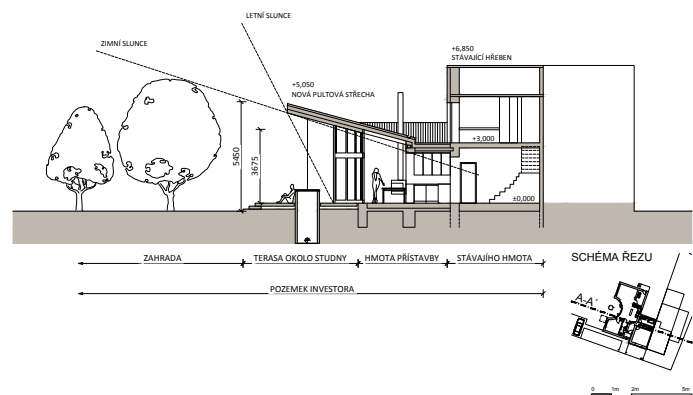
PŘÍČNÝ ŘEZ A DISPOZICE
